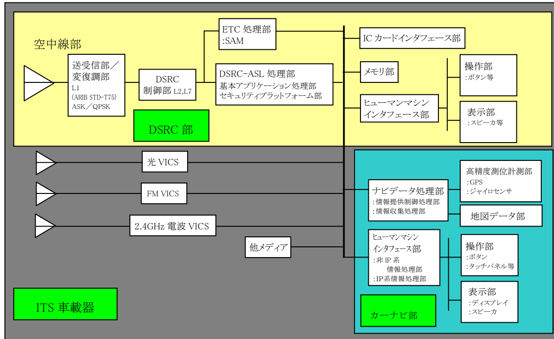
ITS 車載器の機能ブロック図例
