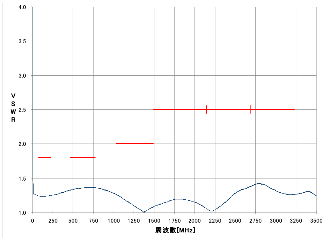
入力VSWR
