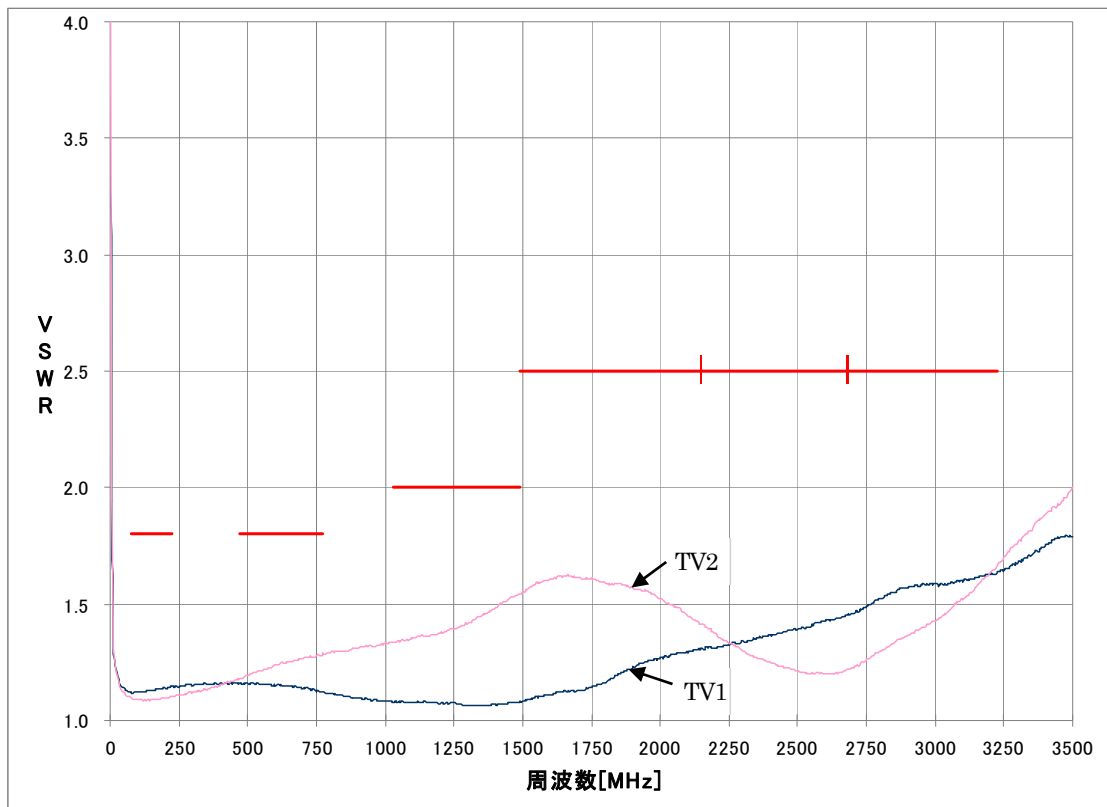
出力VSWR
