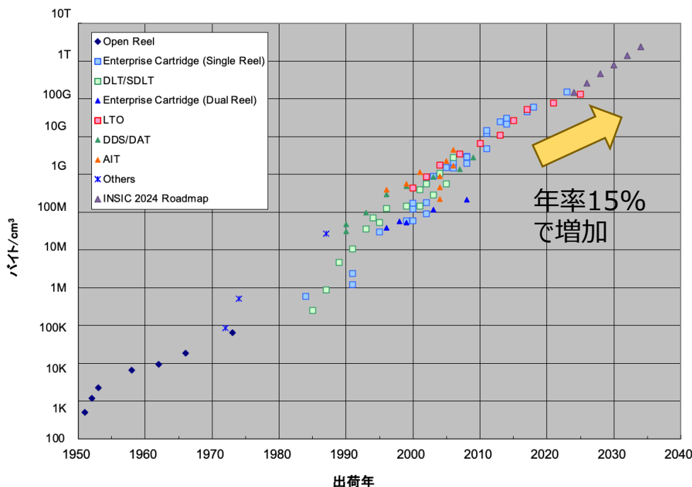
テープカートリッジの容量(1cm³)あたりのバイト数(データ非圧縮時)
