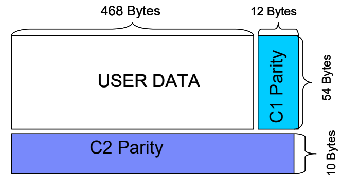
LTO-1の誤り訂正用 ECC
