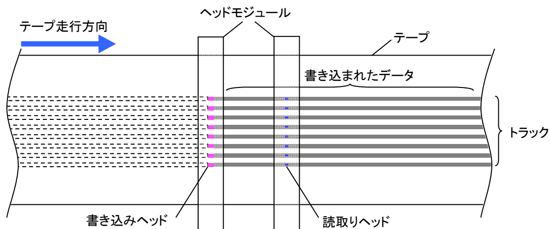
<図1 LTO のヘッド>
