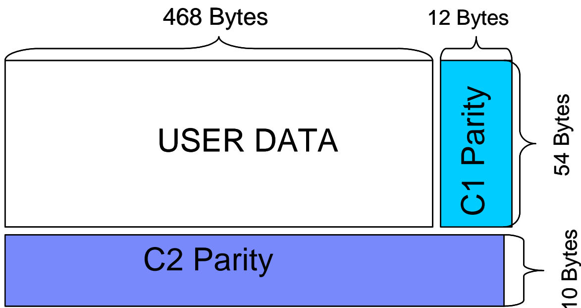
<図3 LTOの誤り訂正用ECC>
