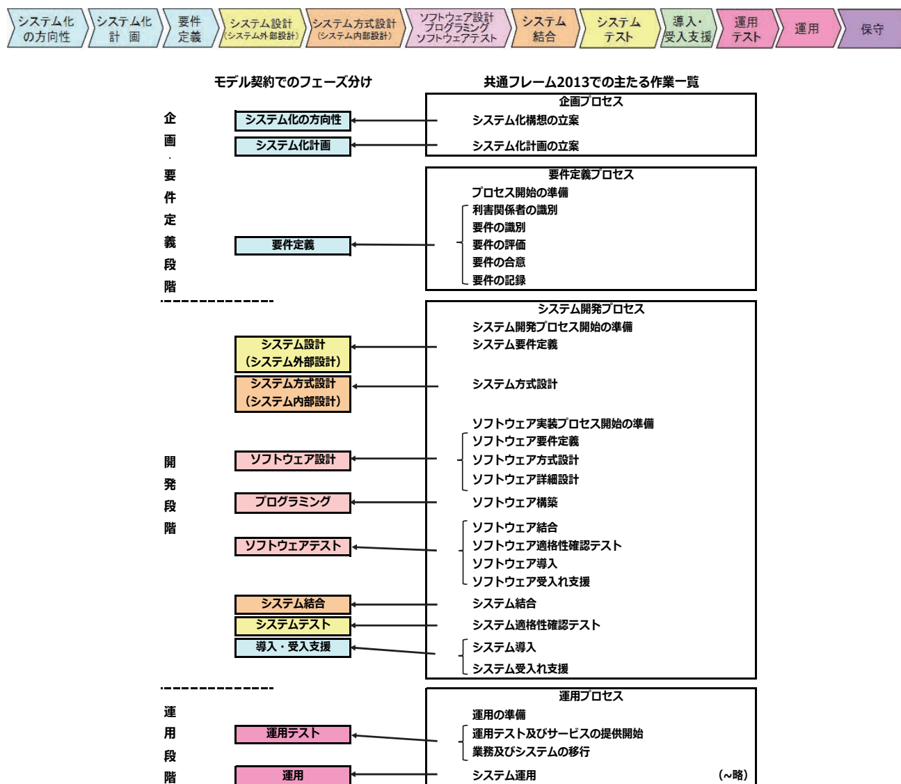
図1 前提とする開発プロセス 6
