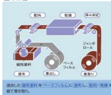
塗布工程
