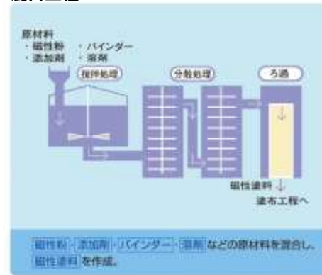
混合工程
